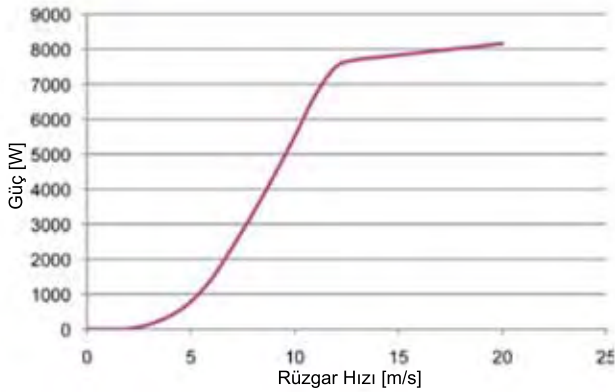
GÜÇ GRAFIĞI
