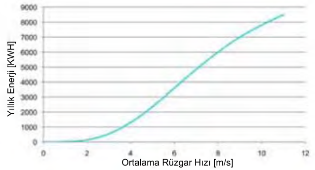
YILLIK ÜRETİM
