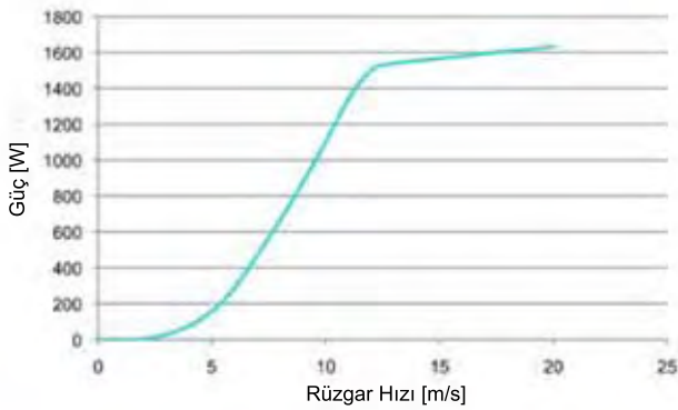
GÜÇ GRAFİĞİ
